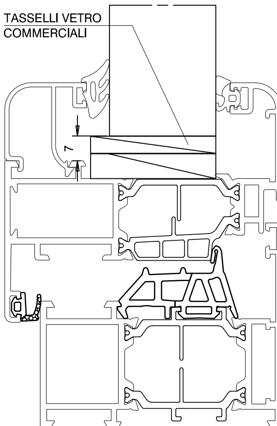
TELAIO MOBILE
