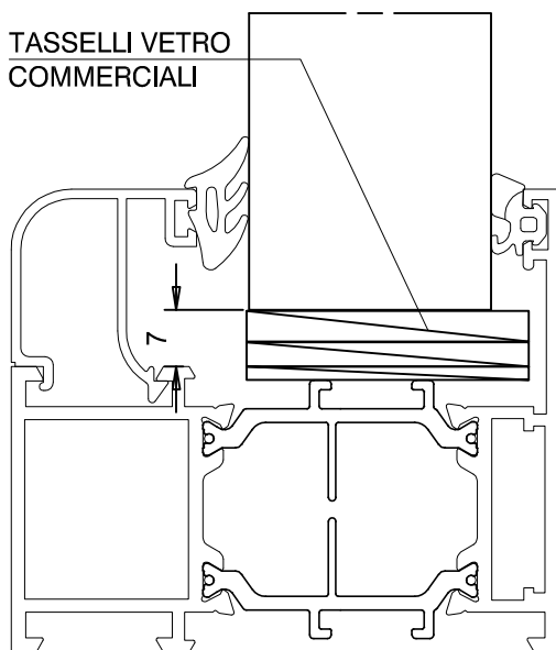
TELAIO FISSO
