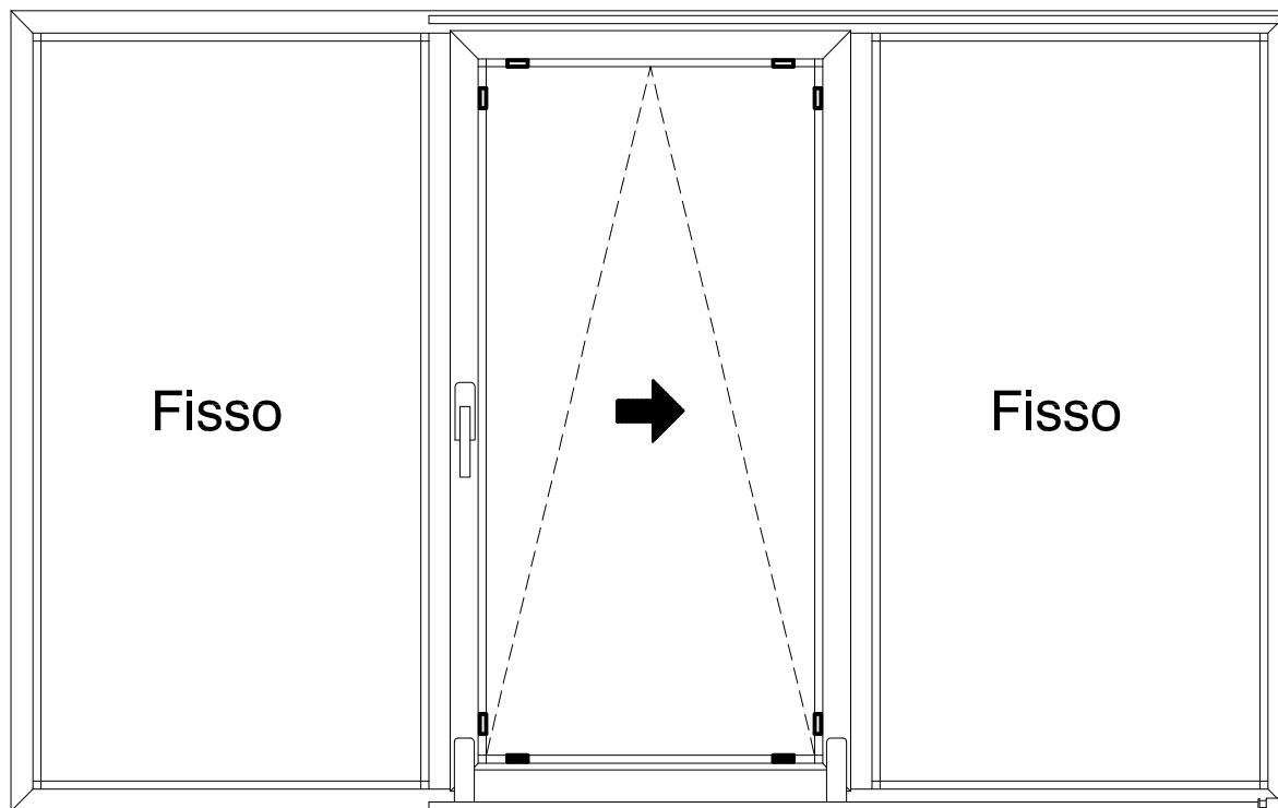
Scorrevole parallelo - schema G
